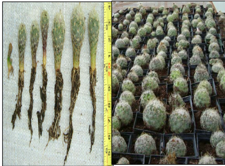
Figura 7. Efecto de Azospirillum sp. en el proceso rizogénico de T. knuthianus (Boed.) John & Riha. Invernadero del Campo Experimental Saltillo CIRNE-INIFAP.
